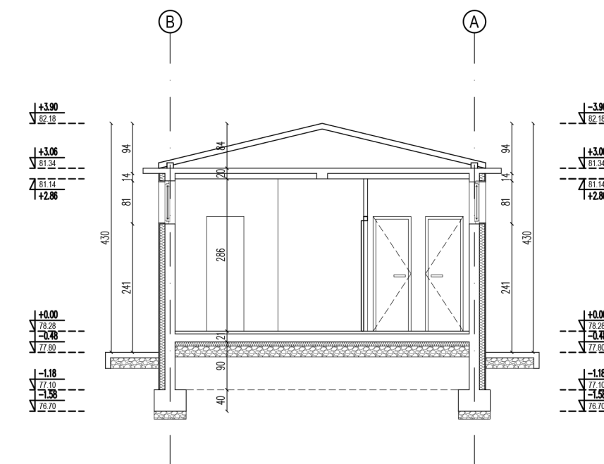
ПРЕСЕК 3-3
