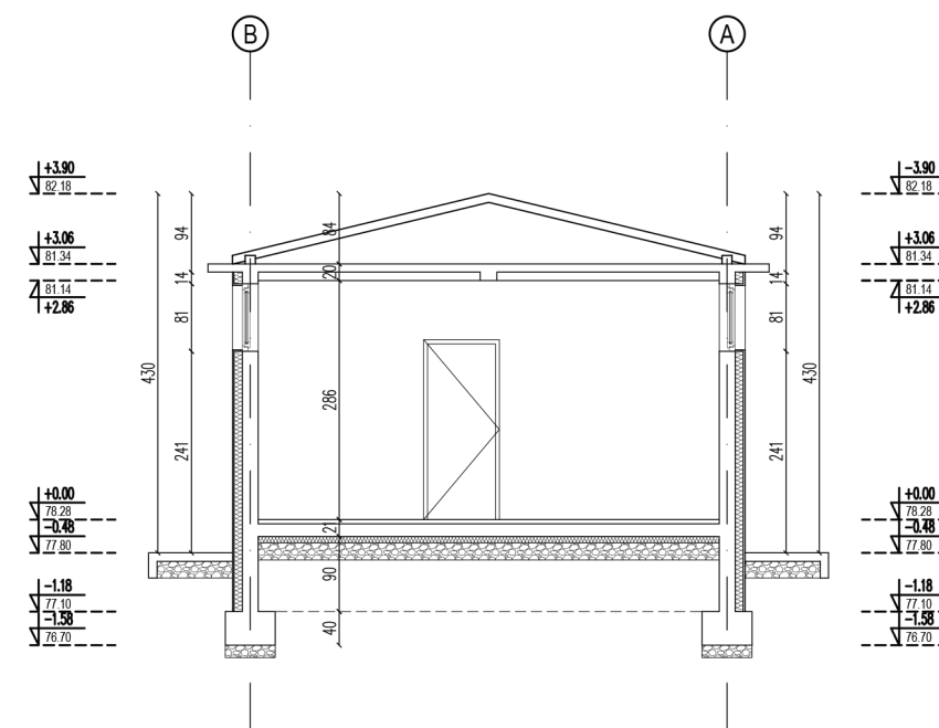
ПРЕСЕК 2-2
