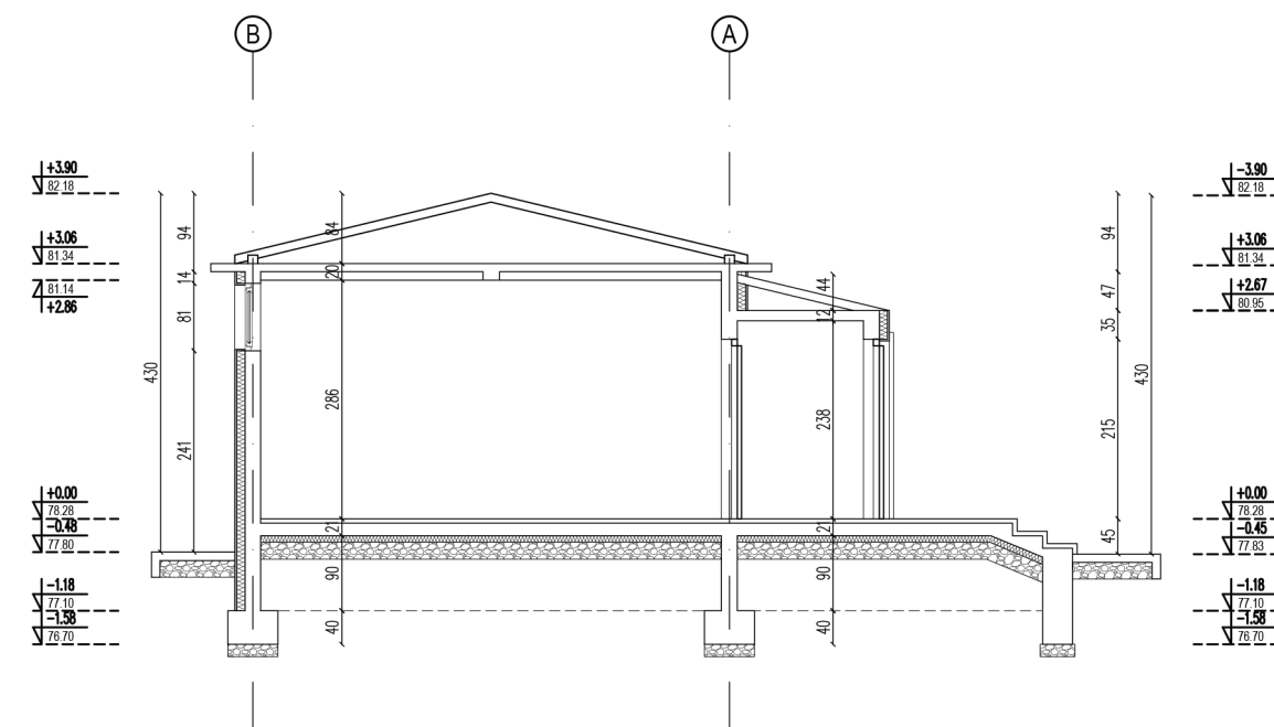
ПРЕСЕК 1-1
