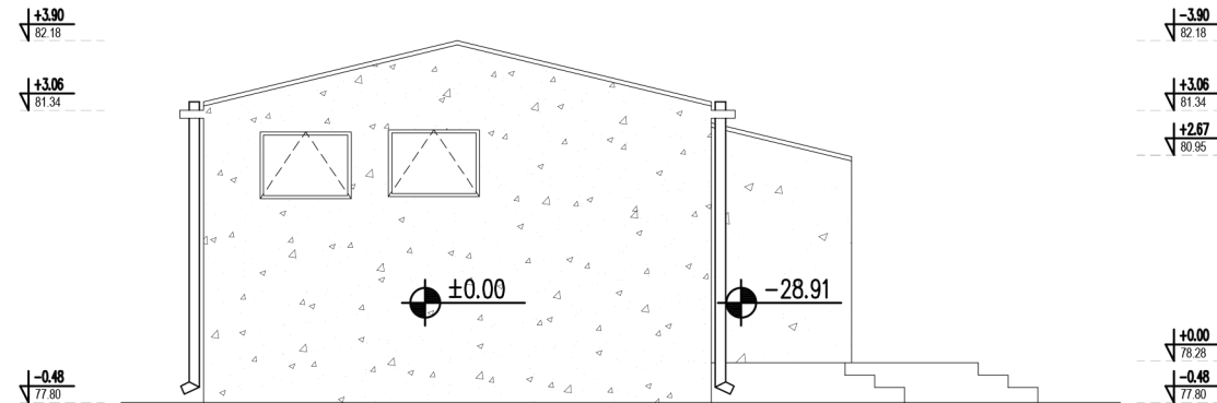
СЕВЕРОЗАПАДНА ФАСАДА
