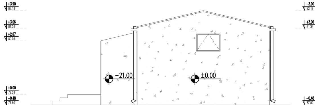
ЈУГОИСТОЧНА ФАСАДА
