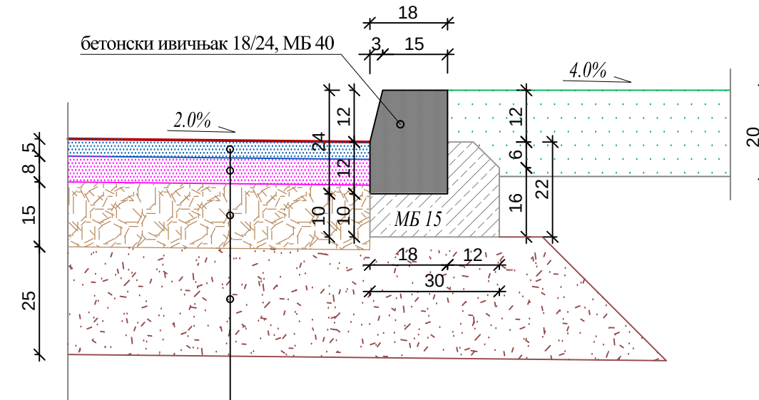
ДЕТАЉ "Б"
