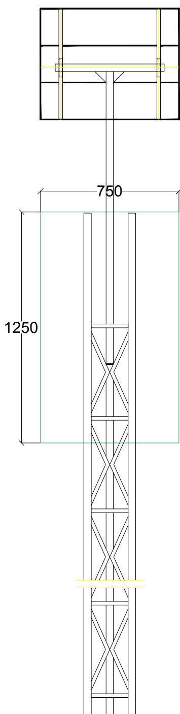
Поглед спреда
