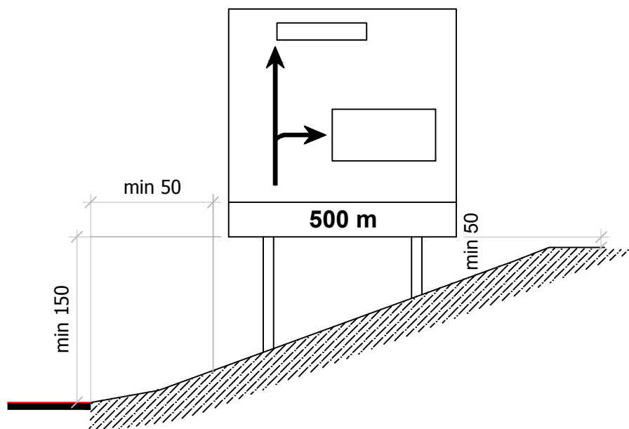
1. Положај табли у усеку
