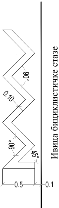
Детаљ обележавања "цик-цак" линије
