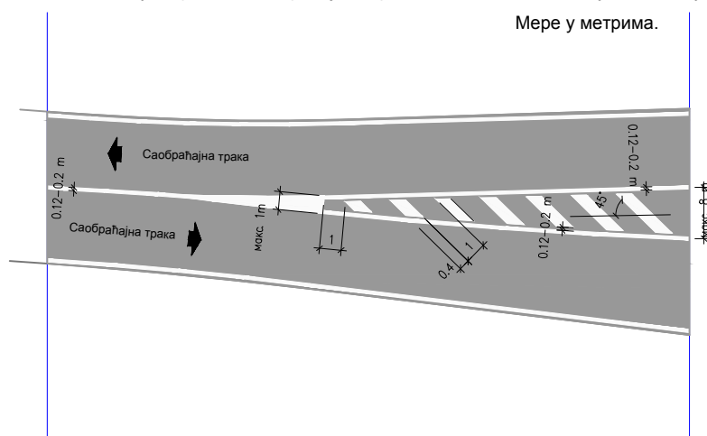
Површина забрањена за саобраћај између две траке са супротним смеровима V \leq 50 \text{ km/h}
