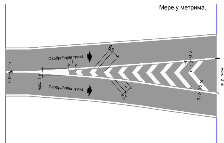
Површина забрањена за саобраћај између две траке са истим смеровима V \leq 50 \text{ km/h}
