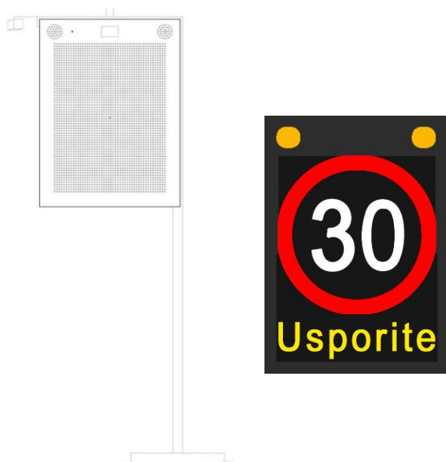
Могући изглед/ конфигурација „лица“ VMS дисплеја
