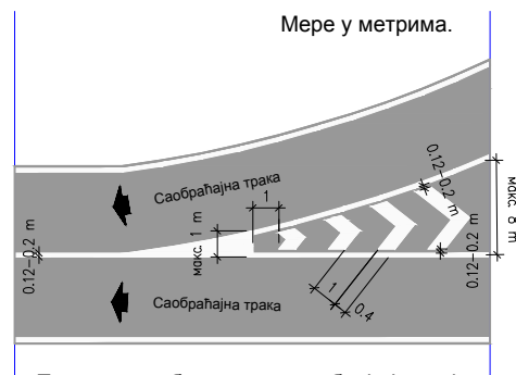
Површина забрањена за саобраћај између две траке са истим смеровима V \leq 50 \text{ km/h}
